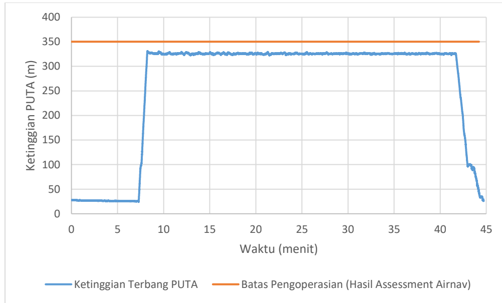
Evaluasi ketinggian PUTA terhadap batas pengoperasian pada penerbangan 17 Januari 2023 di Bangka
