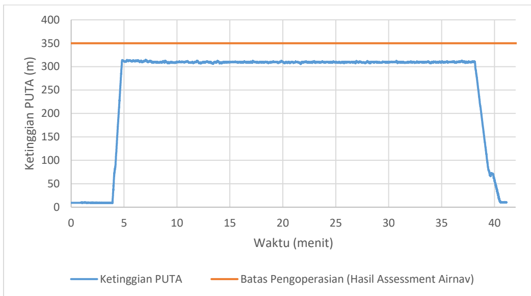
Evaluasi ketinggian PUTA terhadap batas pengoperasian pada penerbangan 2 Februari 2023 pukul 10.08 WIB di Belitung
