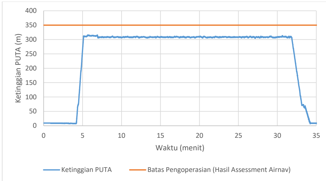
Evaluasi ketinggian PUTA terhadap batas pengoperasian pada penerbangan 1 Februari 2023 pukul 10.00 WIB di Belitung
