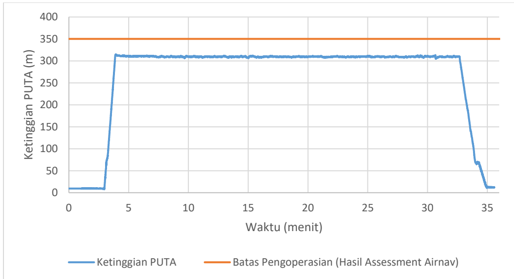
Evaluasi ketinggian PUTA terhadap batas pengoperasian pada penerbangan 2 Februari 2023 pukul 14.00 WIB di Belitung
