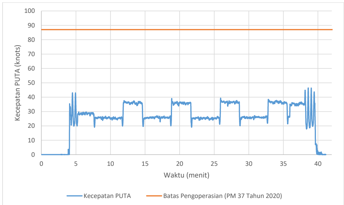
Evaluasi kecepatan PUTA terhadap batas pengoperasian pada penerbangan 2 Februari 2023 pukul 10.08 WIB di Belitung
