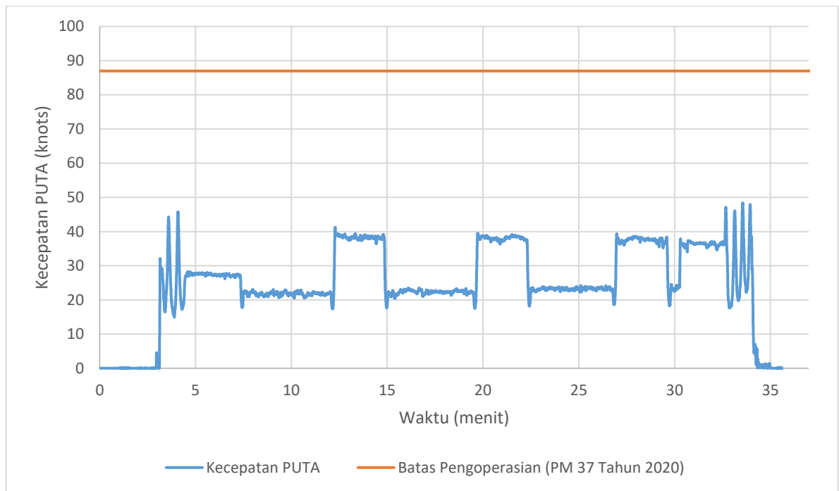
Evaluasi kecepatan PUTA terhadap batas pengoperasian pada penerbangan 2 Februari 2023 pukul 14.00 WIB di Belitung
