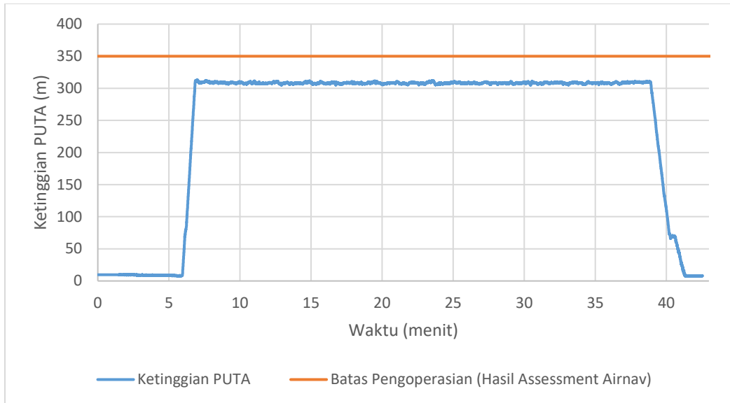
Evaluasi ketinggian PUTA terhadap batas pengoperasian pada penerbangan 2 Februari 2023 pukul 09.22 WIB di Belitung
