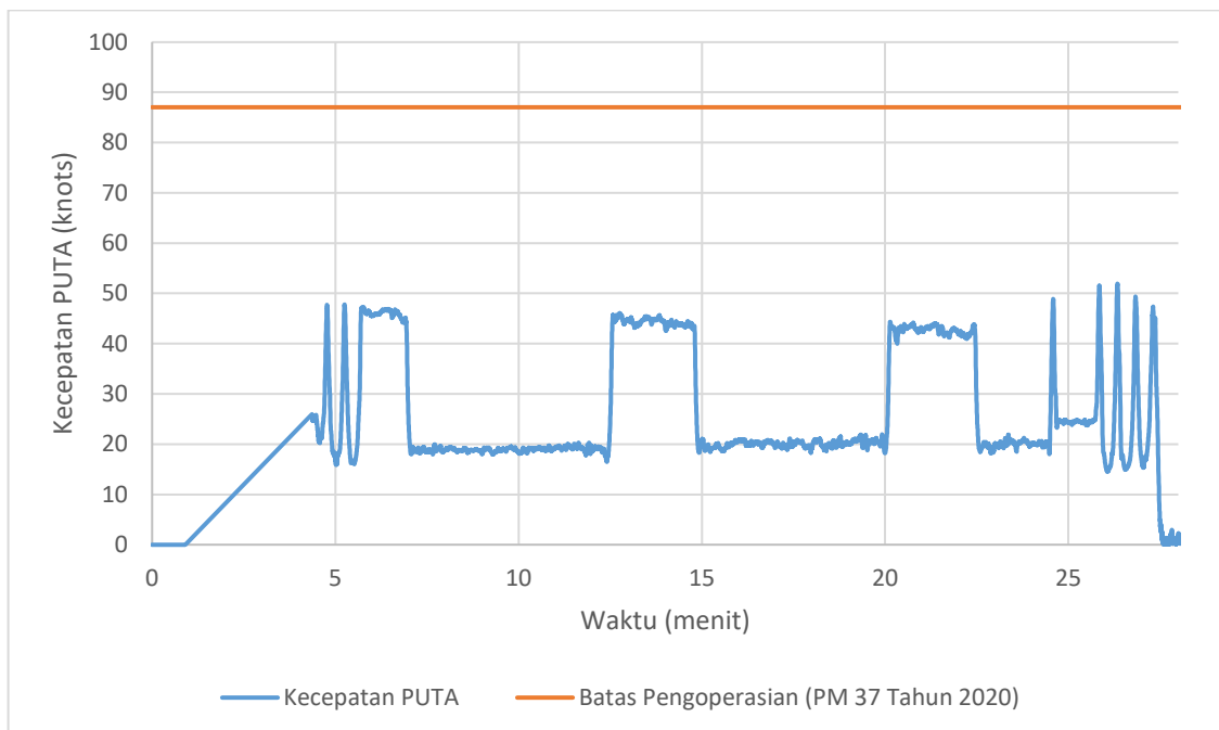
Evaluasi kecepatan PUTA terhadap batas pengoperasian pada penerbangan 1 Februari 2023 pukul 10.43 WIB di Belitung
