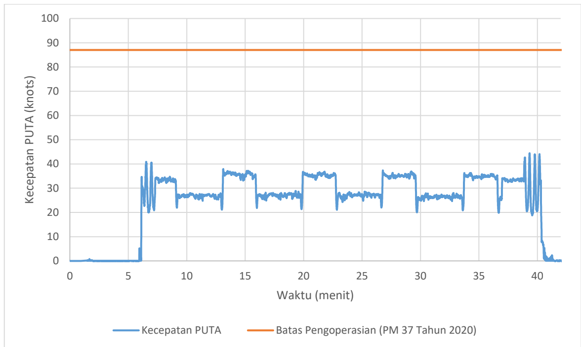
Evaluasi kecepatan PUTA terhadap batas pengoperasian pada penerbangan 2 Februari 2023 pukul 09.22 WIB di Belitung
