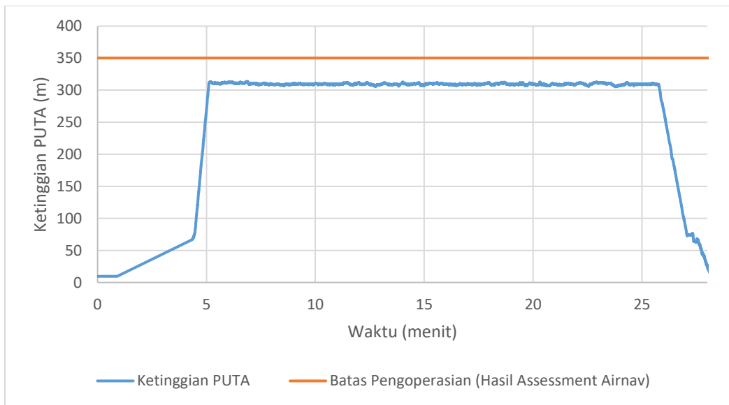
Evaluasi ketinggian PUTA terhadap batas pengoperasian pada penerbangan 1 Februari 2023 pukul 10.43 WIB di Belitung
