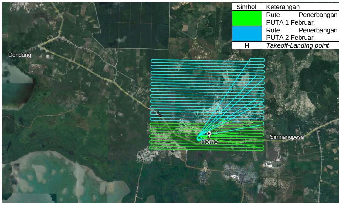
Rute pengoperasian PUTA di Belitung
