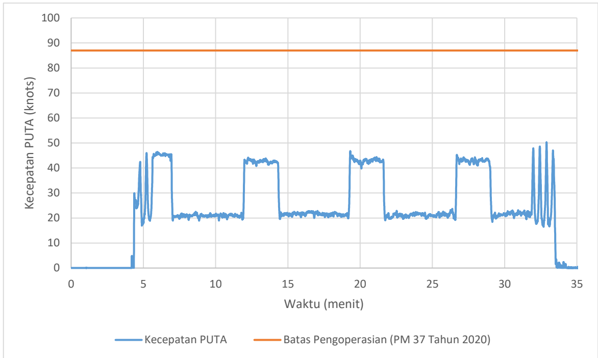
Evaluasi kecepatan PUTA terhadap batas pengoperasian pada penerbangan 1 Februari 2023 pukul 10.00 WIB di Belitung
