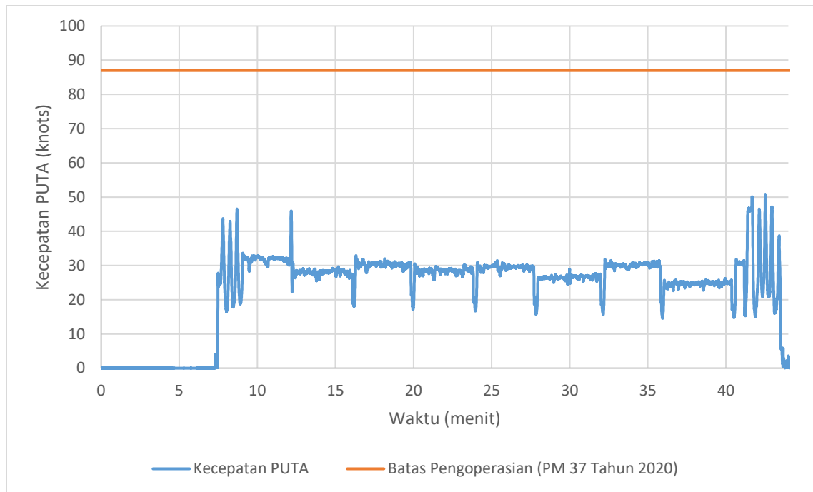
Evaluasi kecepatan PUTA terhadap batas pengoperasian untuk penerbangan 17 Januari di Bangka
